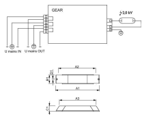
Tekniset tiedot Philips HID-PV m 35 / I CDM 220-240V 50/60Hz
